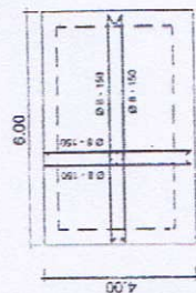
DETAIL PENULANGAN LANTAI OLAK
