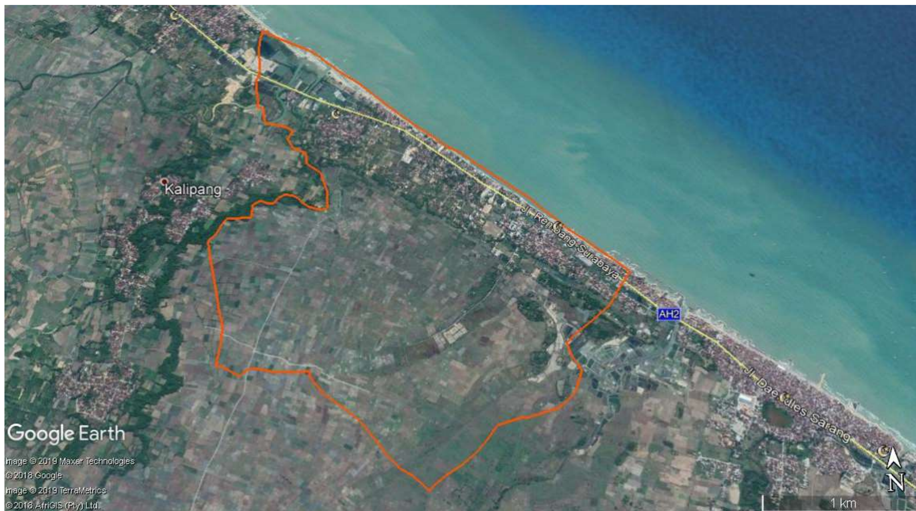
Gambar 1 Peta Lokasi Rencana Ls. Kalipang di Desa Kalipang, Kecamatan Sarang, Kabupaten Rembang
