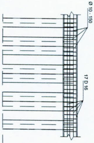
DETAIL PENUNGGAN PILE CAP Skala 1 : 50
