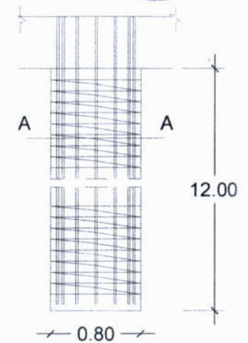
DETAIL PENULANGAN BOR PILE SKALA D,
