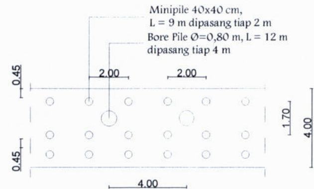
DENAH PEMANCANGAN Mini Pile Dan Bor Pile SKALA B,
