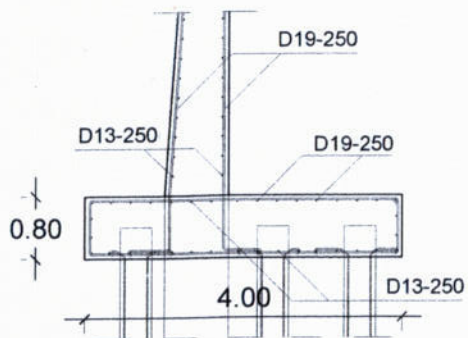
DETAIL PENULANGAN MINI PILE DAN DINDING PENAHAN TANAH SKALA C,
