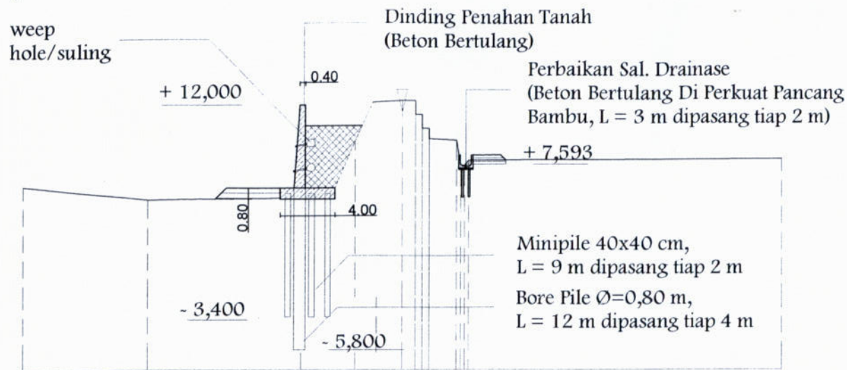
POTONGAN MELINTANG SKALA A
