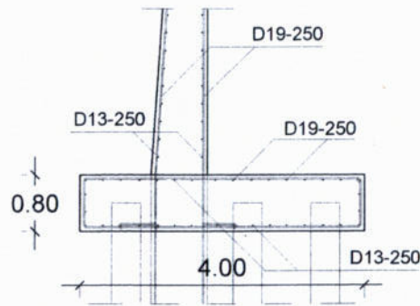
DETAIL PENULANGAN BOR PILE DAN DINDING PENAHAN TANAH SKALA C,
