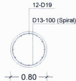
POTONGAN A-A SKALA D,
