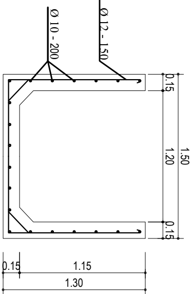
PEMESIAN GOT MIRING Skala 1 : 25
