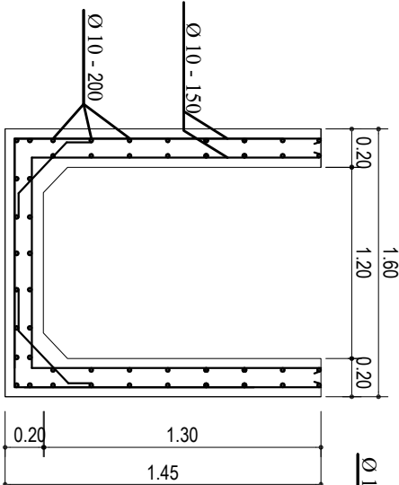
PEMESIAN POT I-I Skala 1 : 25
