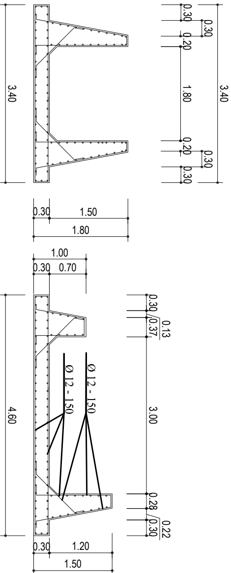
PEMBESIAN POT G-G
