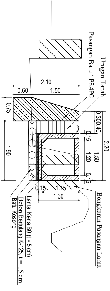
POT E-E Skala 1 : 50
