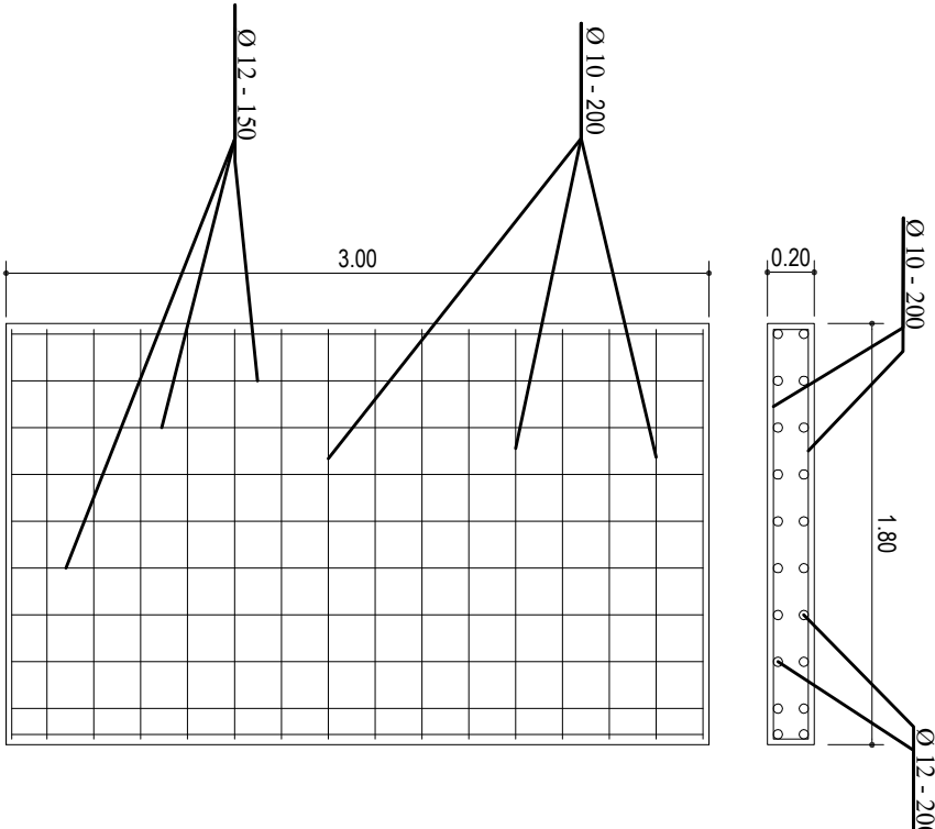
PEMBESIAN POT D-CL Skala 1 : 25
