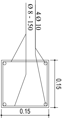
PEMESIAN BALOK TARIK Skala 1 : 50
