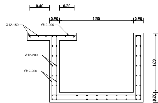
PENULANGAN POT. B-B
