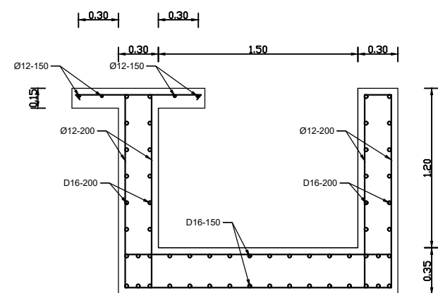
PENULANGAN POT. A-A
