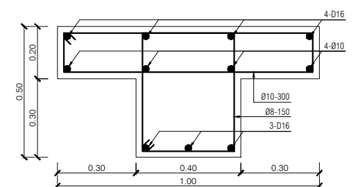
Potongan iv-iv Skala F
