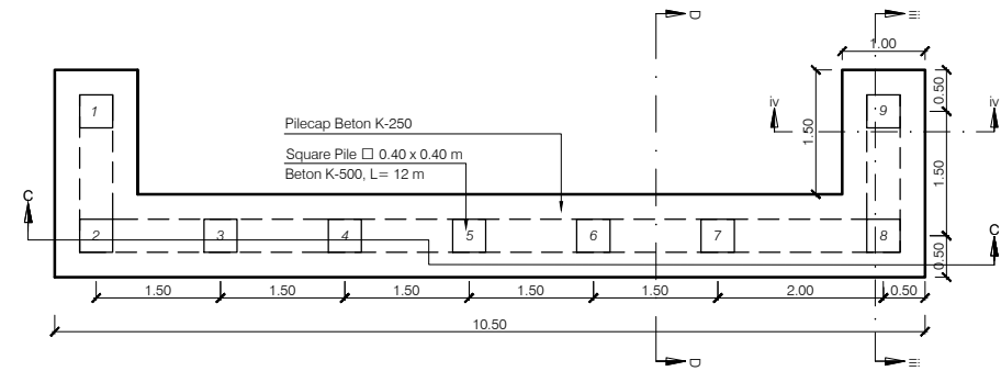
Tampak Atas Krib Skala C
