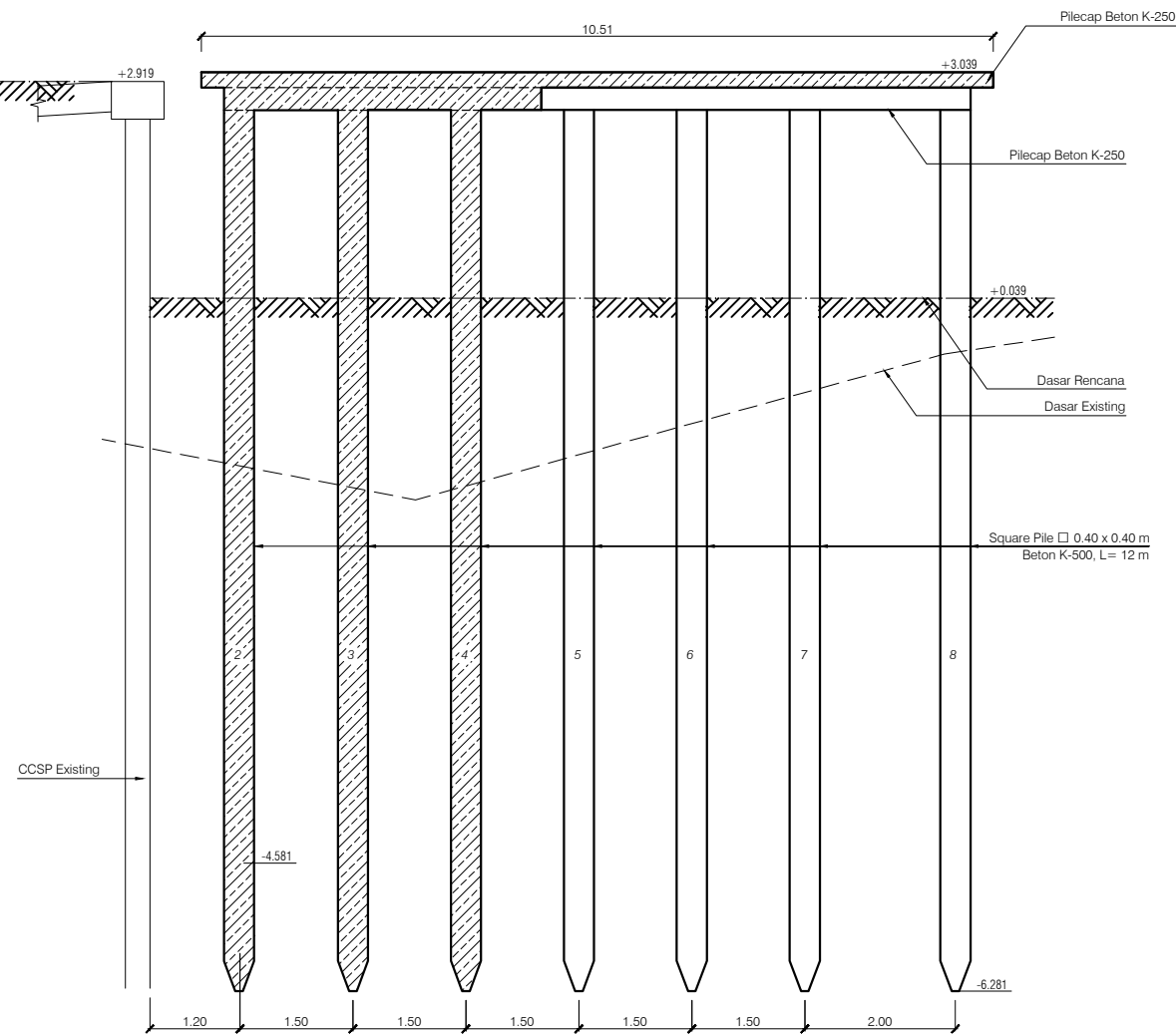
Potongan C-C Skala C
