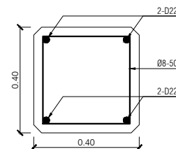
Potongan vi-vi Skala F
