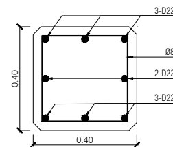
Potongan v-v Skala F
