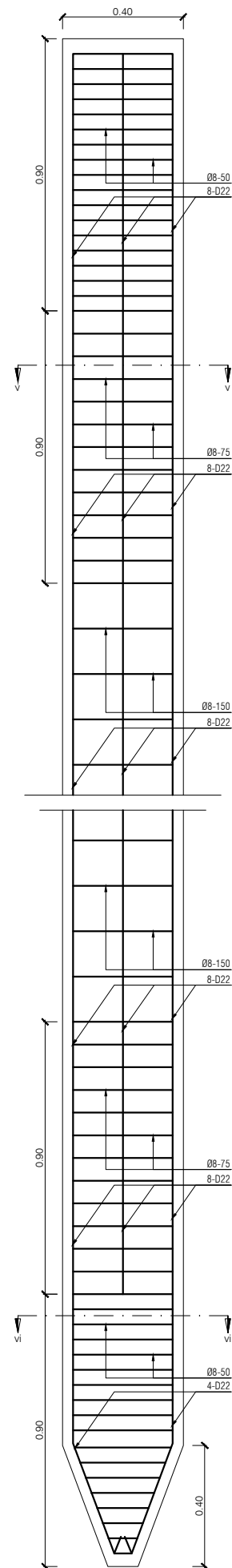
Detail Penulangan Pancang Skala F
