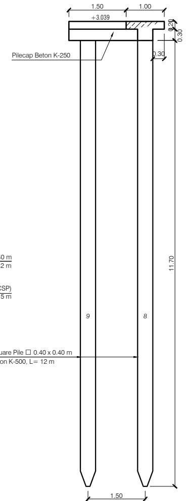
Potongan D-D Skala C
