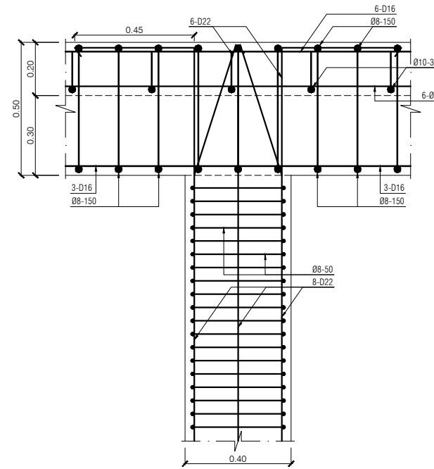
Potongan i-i Skala F
