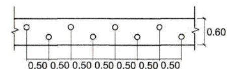
DENAH PANCANG BAMBU Skala 1 : 50
