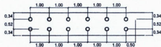
DENAH PANGCANG BAMBU Skala 1 : 40
