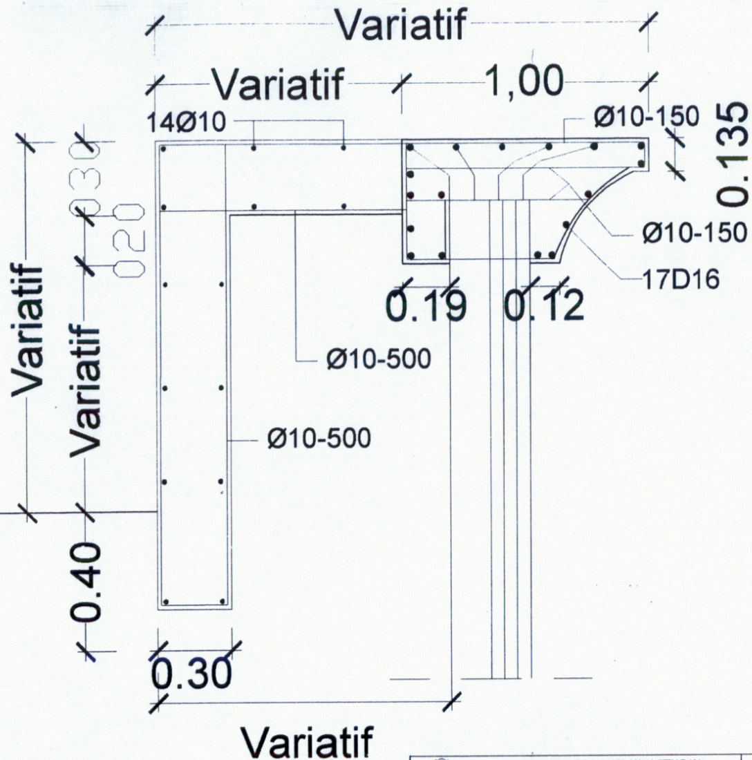
STR 01 DETAIL PENULANGAN PILE CAP SKALA 1:100
