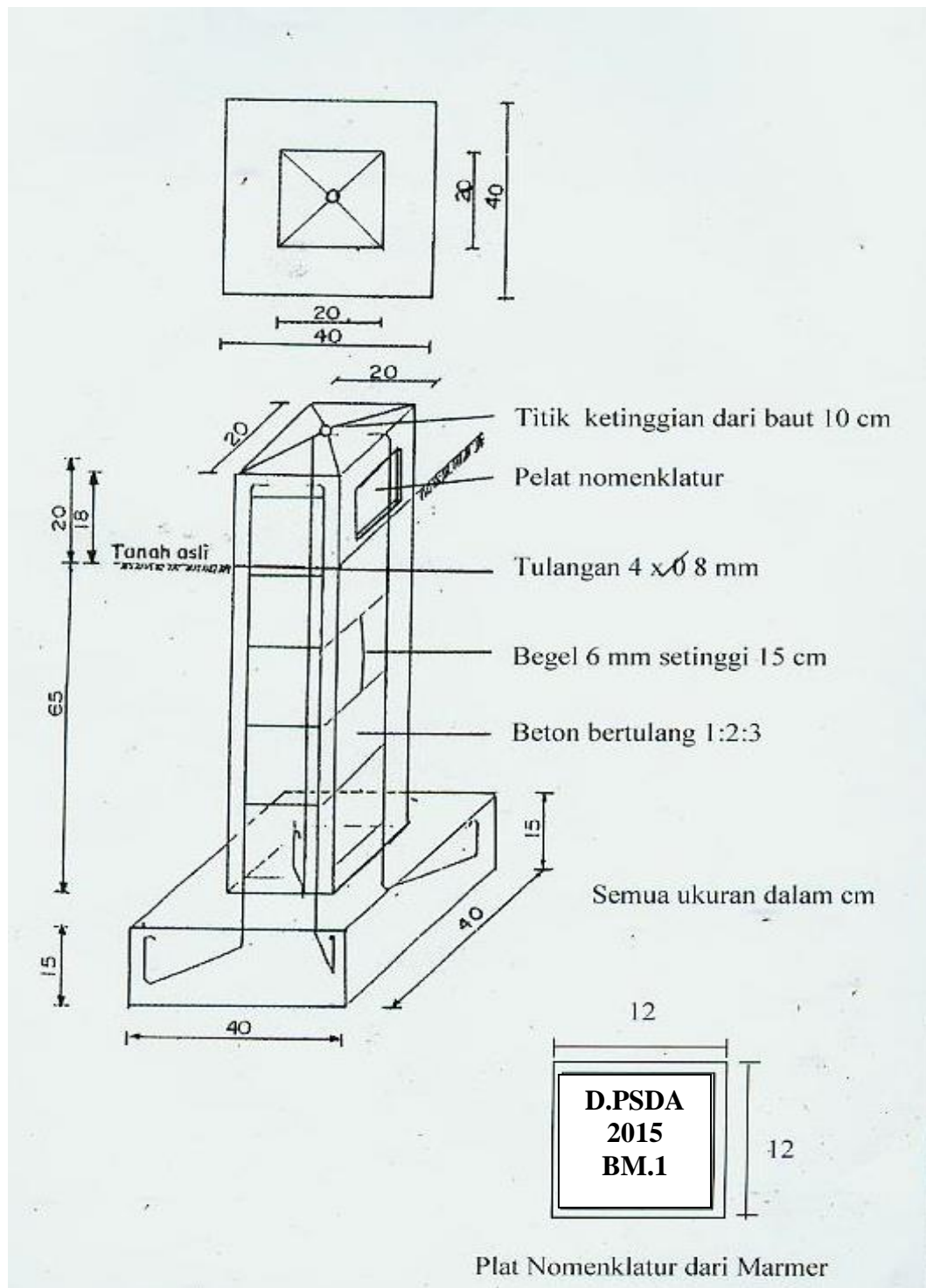
Gambar 1. Spesifikasi Patok BM
